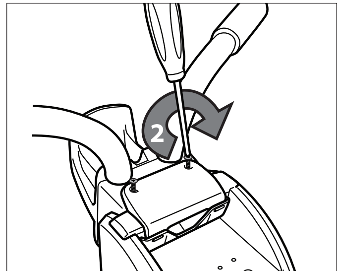
Figura 14. Sujetando la placa de fijación
