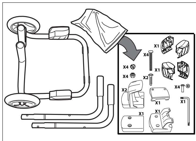
Figura 1. Componentes del Limpiafondos Sección 3. Armado y uso inicial
