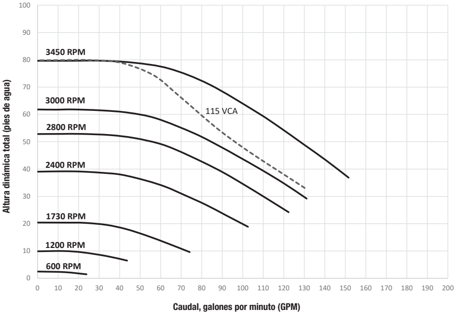
Curvas de desempeño de VSSHP220DV2A(S)
