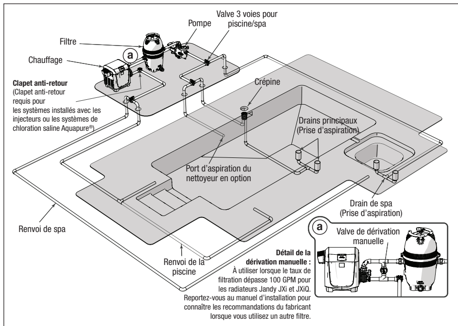
Figure 3. Installation de la tuyauterie typique
