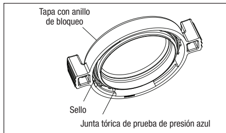
Figura 14. Junta tórica de prueba de presión azul
