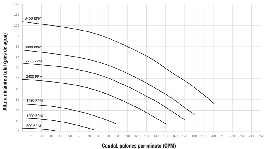
Curvas de desempeño de VSSHP3802A(S)
