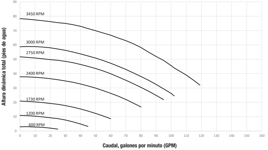
Curvas de desempeño de VSSHP220DV2A(S)
