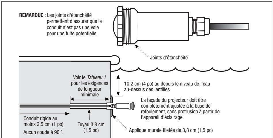
Figure 2. Installation standard avec une applique murale de 3,8 cm (1,5 po) pour piscine
